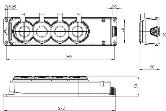
Колодка 4-местная с защитными крышками каучуковая
