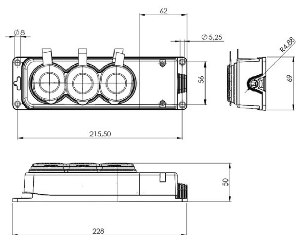
Колодка 3-местная с защитными крышками каучуковая
